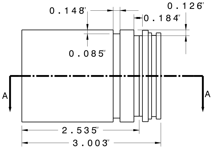
Right view Scale: 1:1
