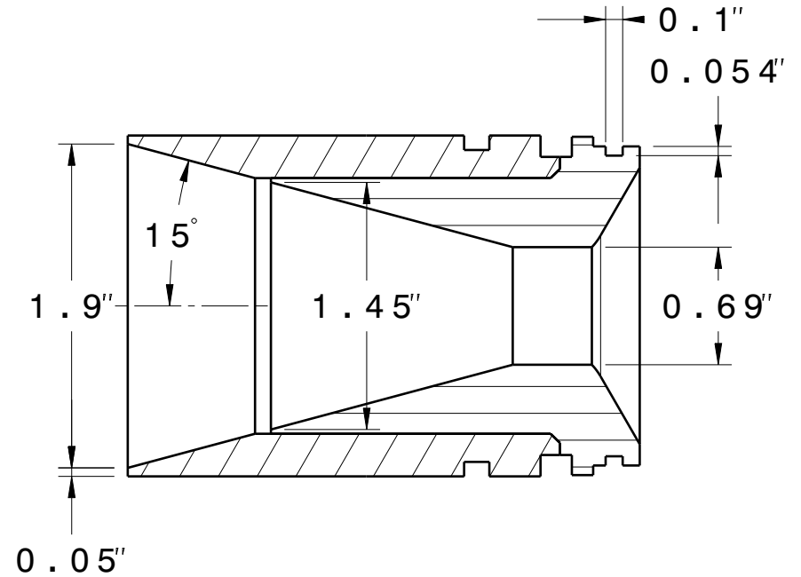
Section view A-A Scale: 1:1
